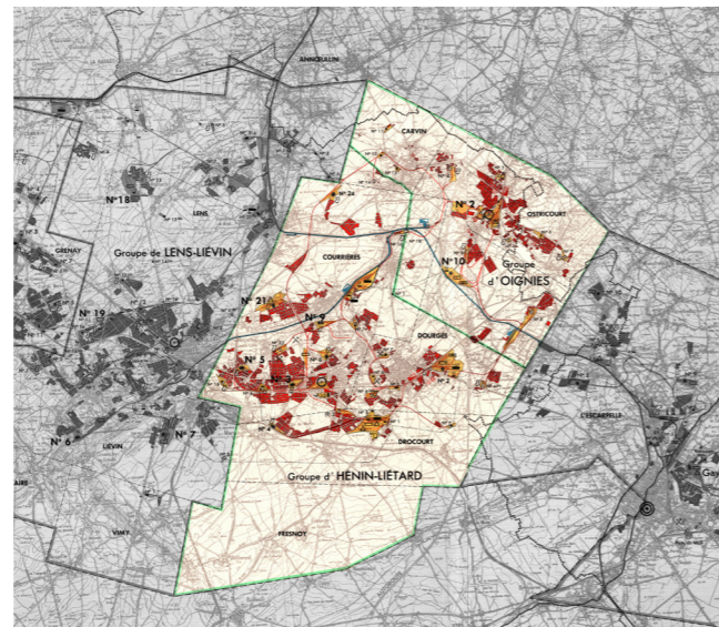
# Cartographie HBNPC - 1964 Groupes d'Hénin-Liétard et Oignies
